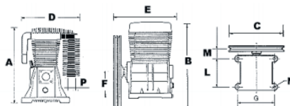
DIMENSIONES
